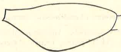
FIG. 1. — Ectemnius (Apoctemnius) saxatilis (CAMERON) ♂ : fémur I vu dorsalement (25 ×).
