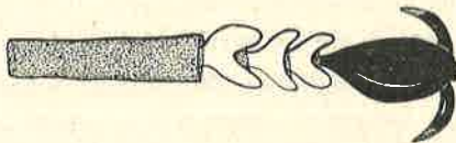
FIG. 2. — Ectemnius (Apoctemnius) saxatilis (CAMERON) ♂ : tarse I (25 ×).
